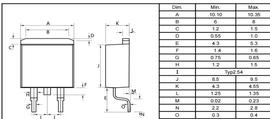
TO-263
